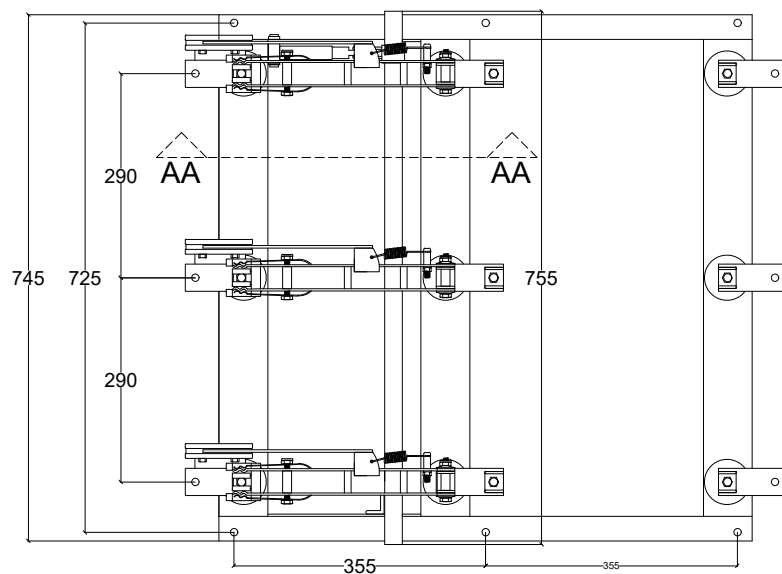
CORTE AA
